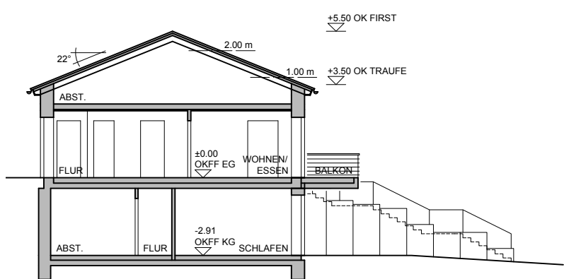
NORDANSICHT
