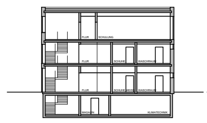
QUERSCHNITT
