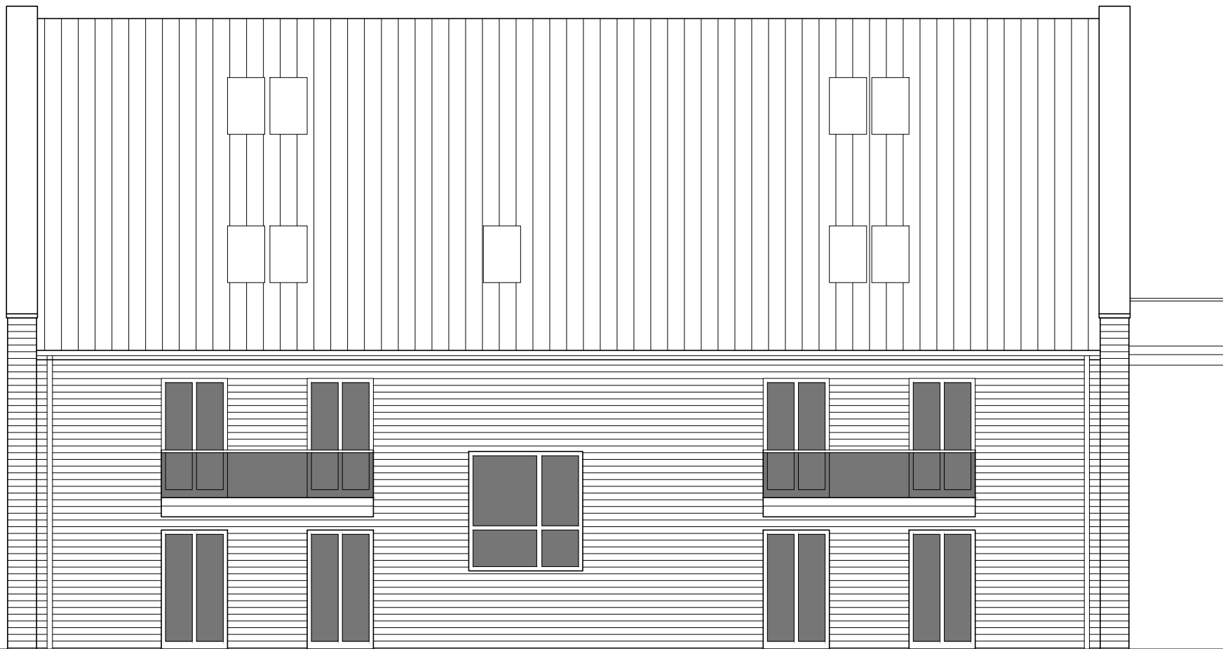
ANSICHT SÜDWEST (GARTEN)
