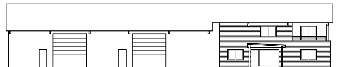
SÜDANSICHT
