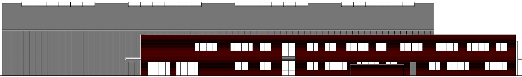
SÜDWESTANSICHT
