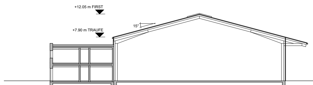
QUERSCHNITT
